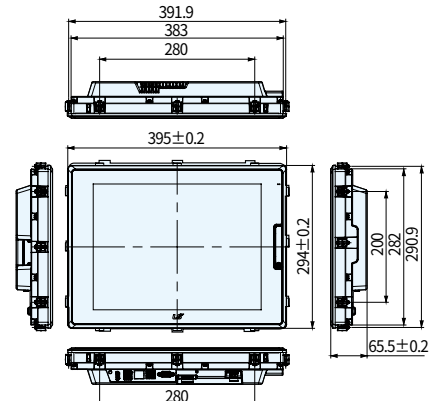
iXP2-1500
