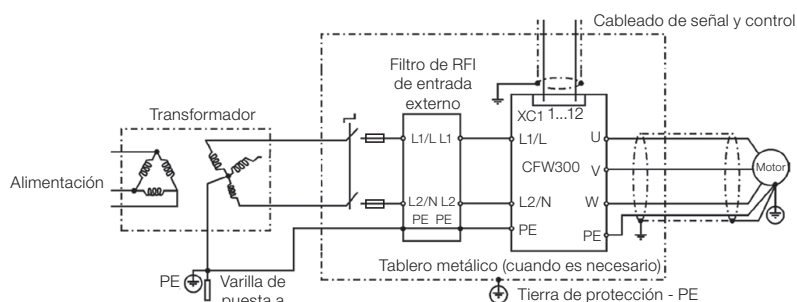
(a) Conexión del filtro RFI monofásico
