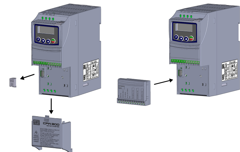
(a) Removal of the protection cover of the connection of the IO expansion accessory (a) Remoción de la tapa de protección de la conexión de los accesorios de expansión de IO's (a) Remoção da tampa de proteção da conexão dos acessórios de expansão de IO's
