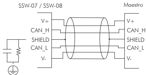
Figura 1 - Conexión DeviceNet
