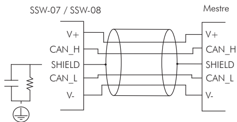
Figura 1 - Conexão DeviceNet
