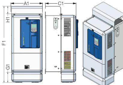
Frame size E 180 and 211 A with Nema1 kit Tamaño E 180 y 211 A con kit Nema1 Mecânica E 180 e 211 A com kit Nema1
