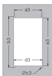
(b) Flange mounting (b) Montaje en flange (b) Montagem em flange
