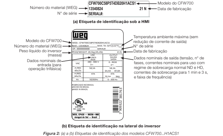
Figura 2: (a) a (b) Etiquetas de identificação dos modelos CFW700...H1ACS1
