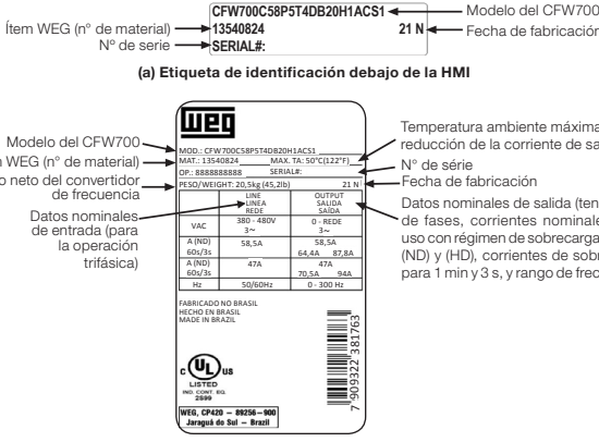
Figura 2: (a) a (b) - Etiquetas de identificación de los modelos CFW700...H1ACS1
