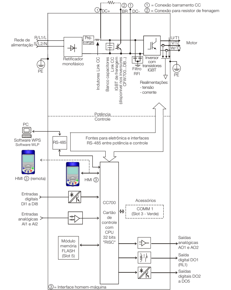
Figura 1: Blocodiagrama do CFW700...modelo H1ACS1
