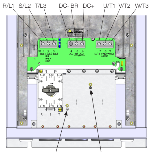
Aterramento Aterramento (d) Mecânica D com grau de proteção IP55
