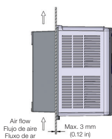
(b) Flange mounting (b) Montaje en flange (b) Montagem em flange
