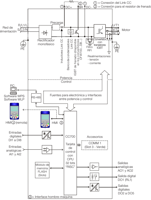
Figura 1: Diagrama de bloques de los modelos CFW700...H1ACS1
