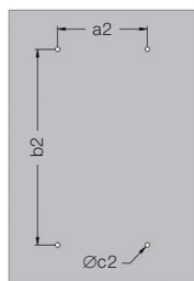
(a) Surface mounting (a) Montaje en superficie (a) Montagem em superfície
