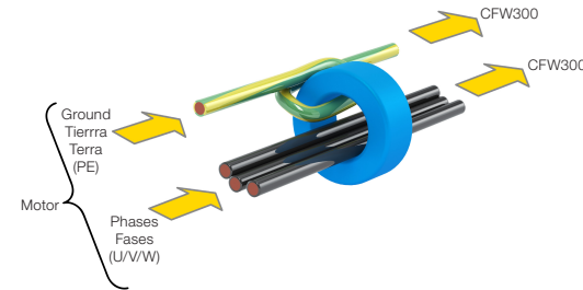
Figure A6: (a) to (d) Common mode choke installation on the motor cables Figura A6: (a) a (d) Instalación del choke de modo común en los cables del motor Figura A6: (a) a (d) Instalação do choke de modo comum nos cabos do motor
