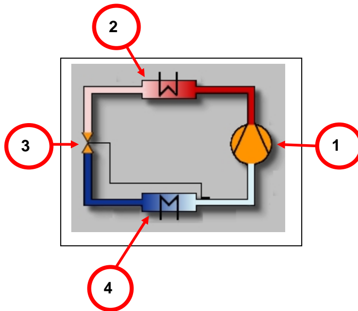
Abbildung 25 – Betriebsschema
