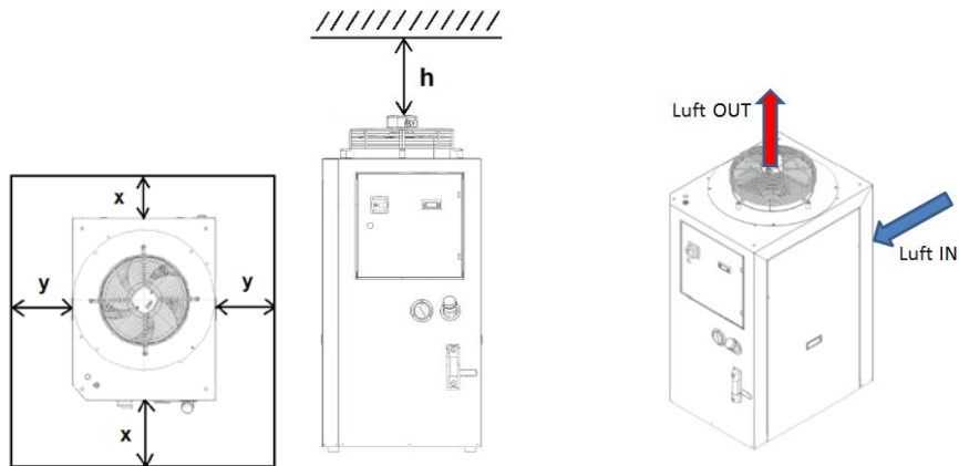
Abbildung 2 – Mindestraumbedarf, x=h=1,5 m; y=0,5 m
