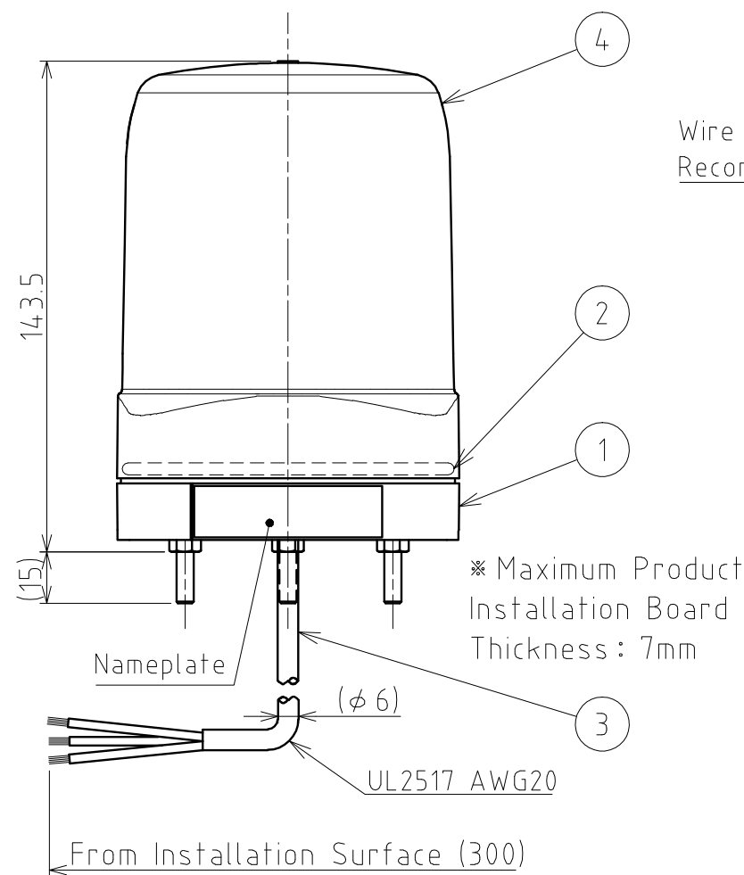
Dimensions
