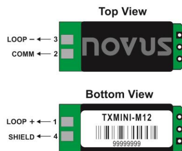
Fig. 3 – Output 4-20 mA
