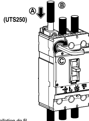
<Fig. 5> wire installation / instalación de cable / installation de fil.
