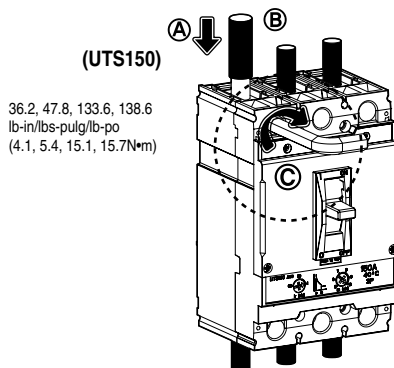
<Fig. 5> wire installation / instalación de cable / installation de fil.
