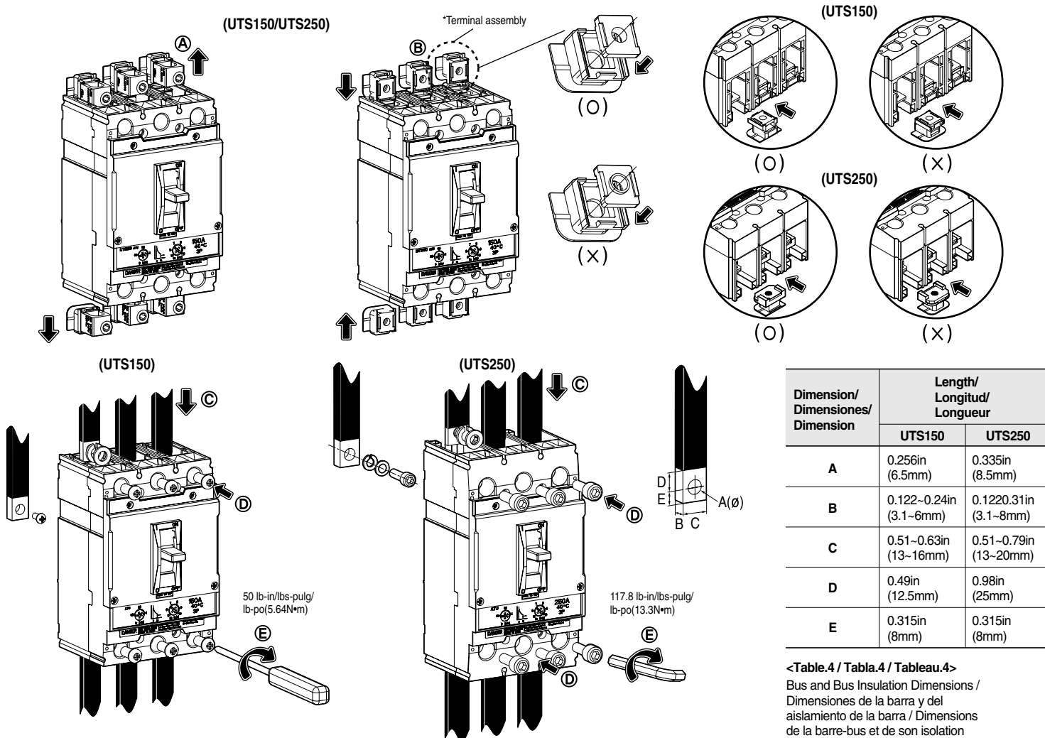
<Fig. 8> bus installation/ Instalación de barras / Installation de bus
