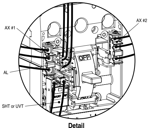
<Fig. 7> Control Wiring Installation / Instalación de cable de control / Installation de câblage de contrôle
