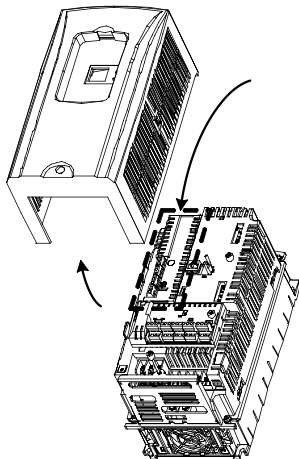
그림 2.1 iS7 위치 제어 전용 엔코더 옵션 장착
