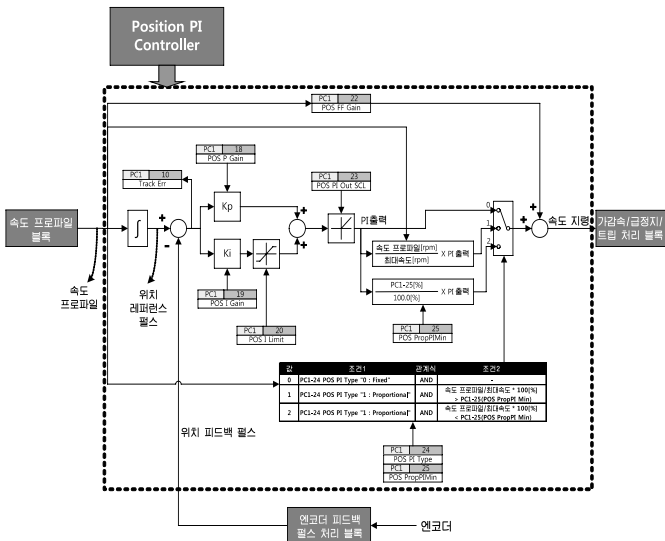
그림 3.4 Position PI Controller 블록도
