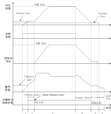
그림 3.8 일반 속도 벡터 제어 Break 동작 그래프
