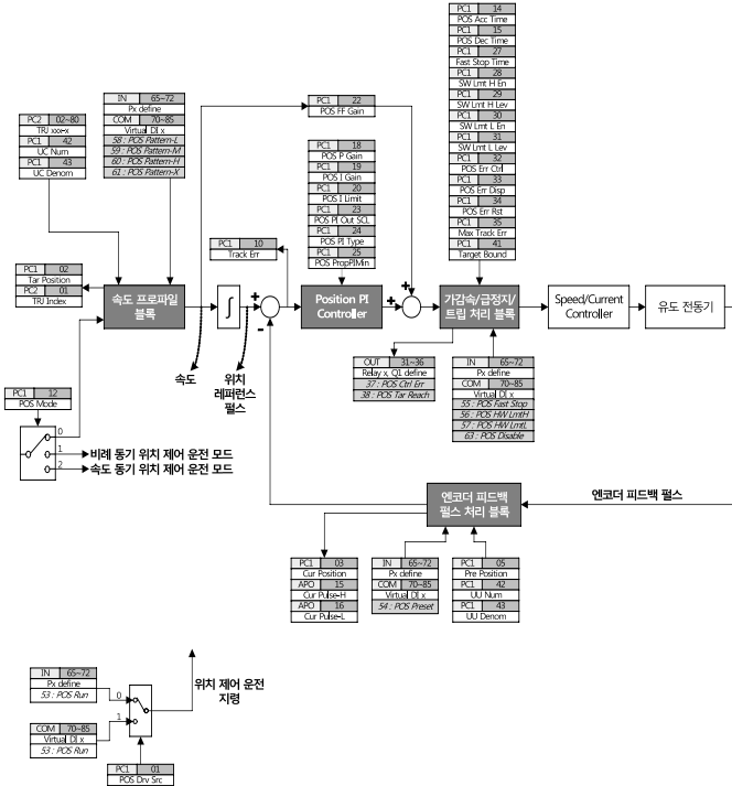
그림 3.1 단독 위치 제어 운전의 전체 블록도
