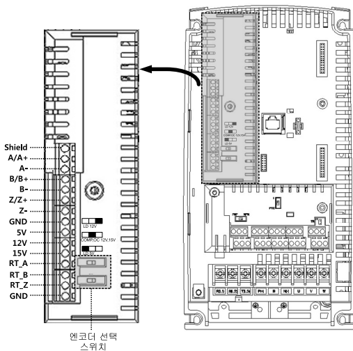
그림 1.1 전체 구성도
