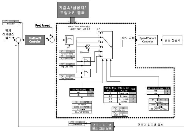
그림 3.5 예외 처리 블록도
