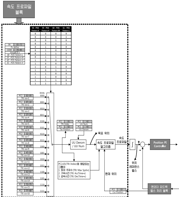
그림 3.2 위치 경로 프로파일 블록
