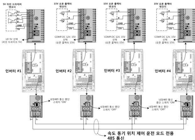
그림 A.4 총 4대 인버터의 속도 동기 위치 제어 운전 결선 방법
