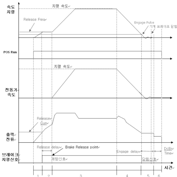
그림 3.7 위치 제어 외부 Break 동작 그래프
