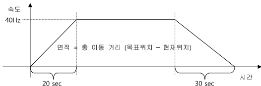
그림 3.3 위치 경로 Reference Pattern
