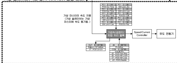
A.2.2.1 속도 동기 위치 제어 운전 모드의 전체 블록도
