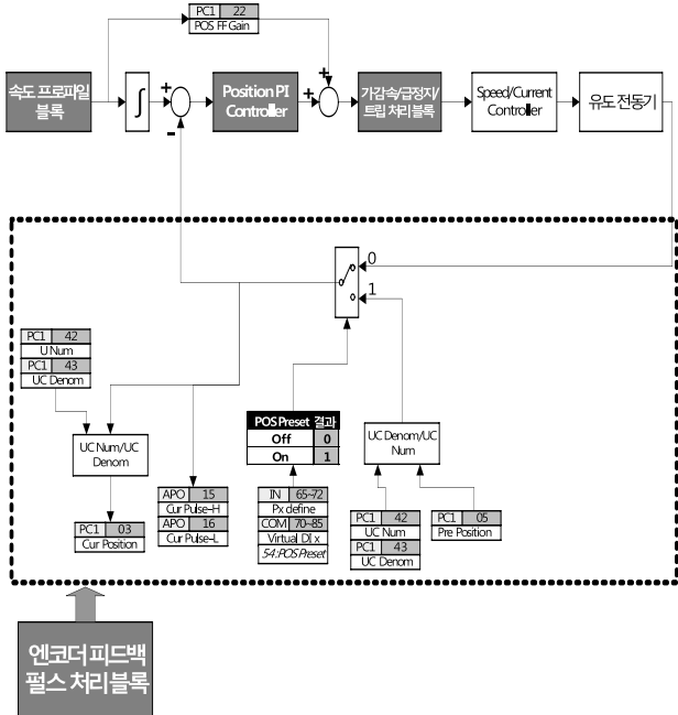
그림 3.6 엔코더 피드백 펄스 처리 블록도
