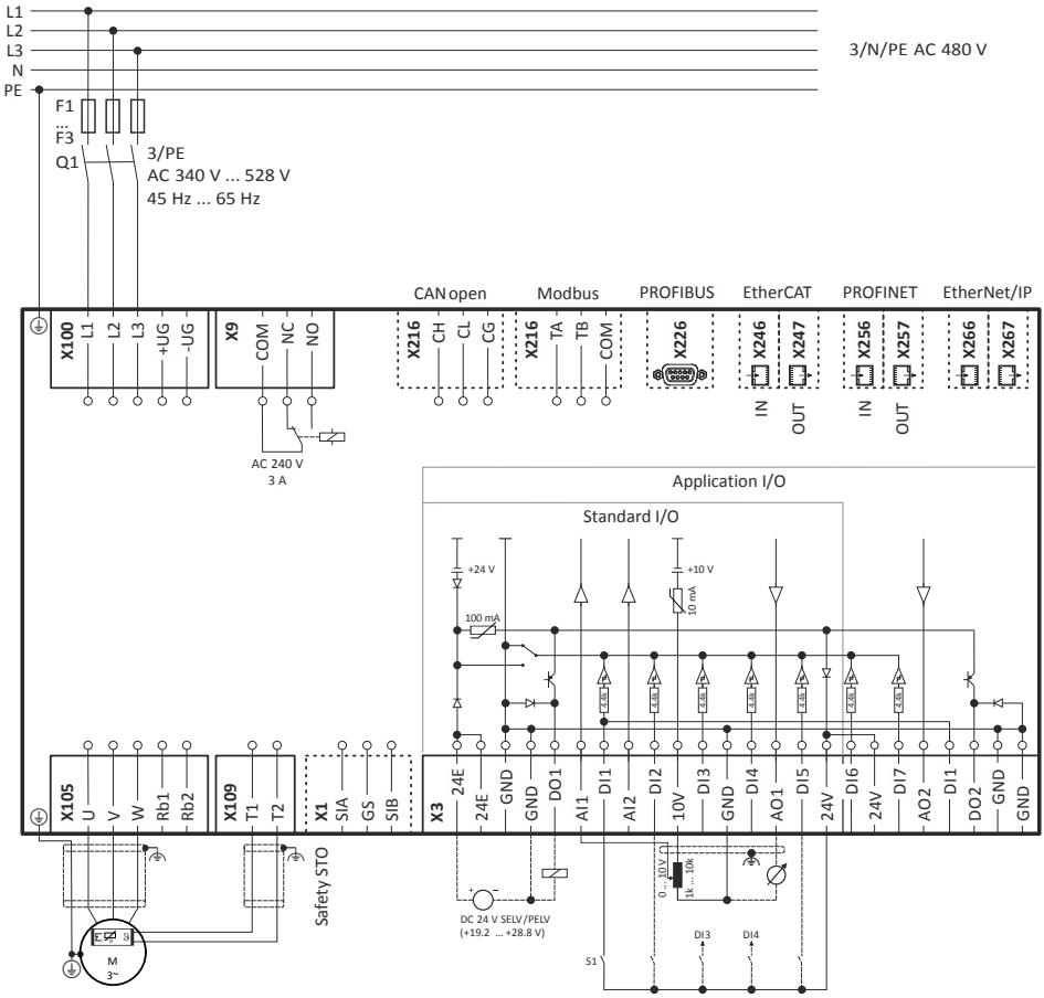
Fig. 1: Wiring example
