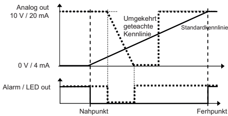
Beispiel für umgekehrt geteachte Kennlinie. 4 mA / 0 V im Fernpunkt, 20 mA / 10 V im Nahpunkt
