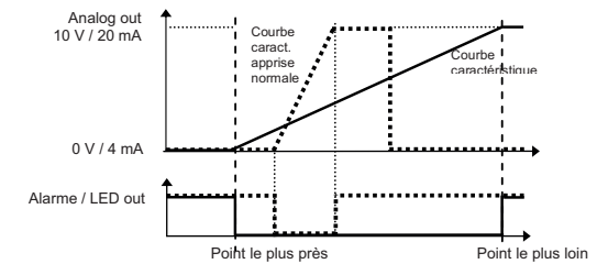
Exemple d'apprentissage d'une courbe caractéristique normale. 4 mA / 0 V point le plus près, 20 mA / 10 V point le plus loin.
